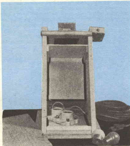
Dettagli costruttivi della stampatrice in tutti i suoi particolari
